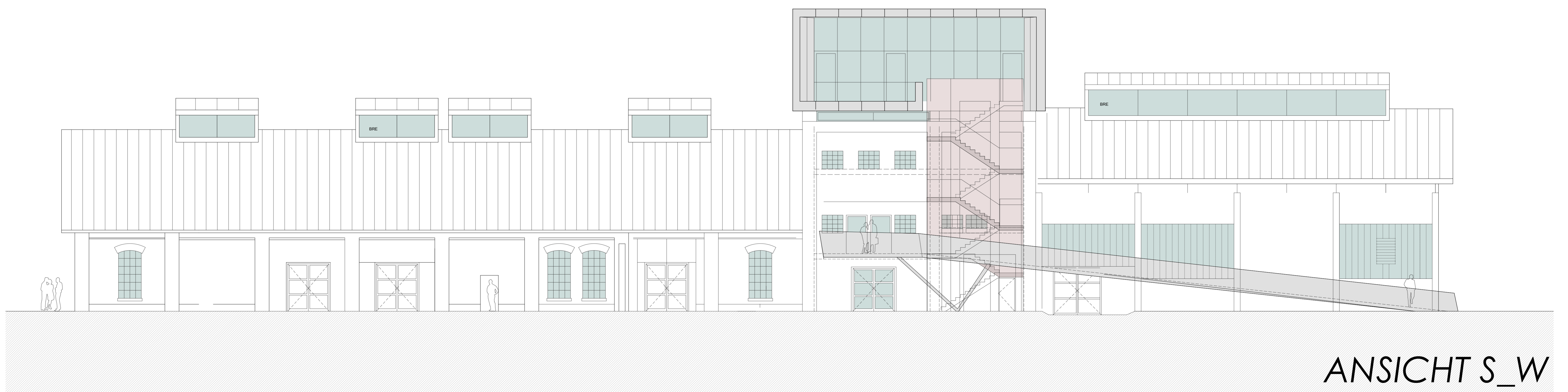
SCHNITT
